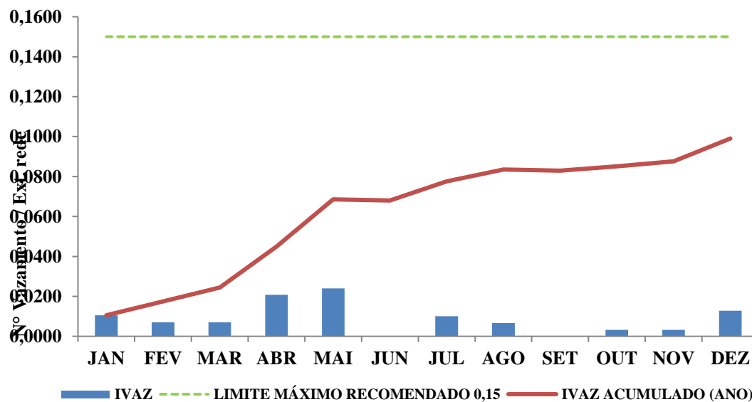
Gráfico 11 - Índice de vazamento no sistema de distribuição de gás (IVAZ)
