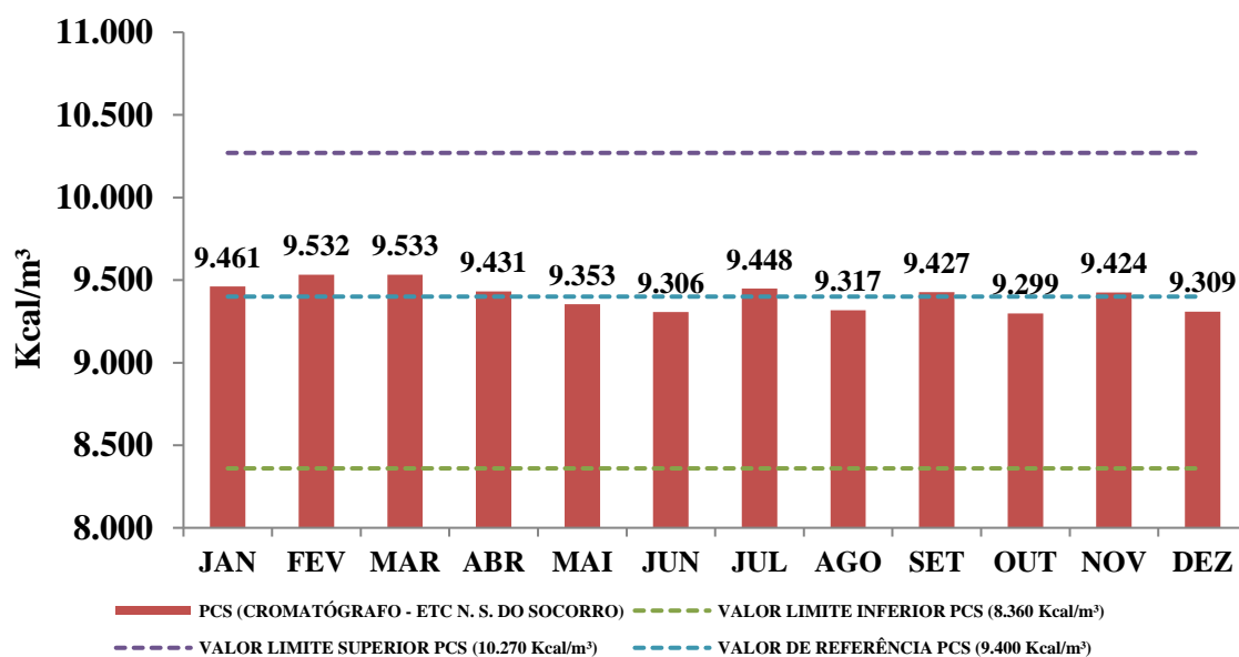
Gráfico 16 - PCS (ETC Nossa Senhora do Socorro)
