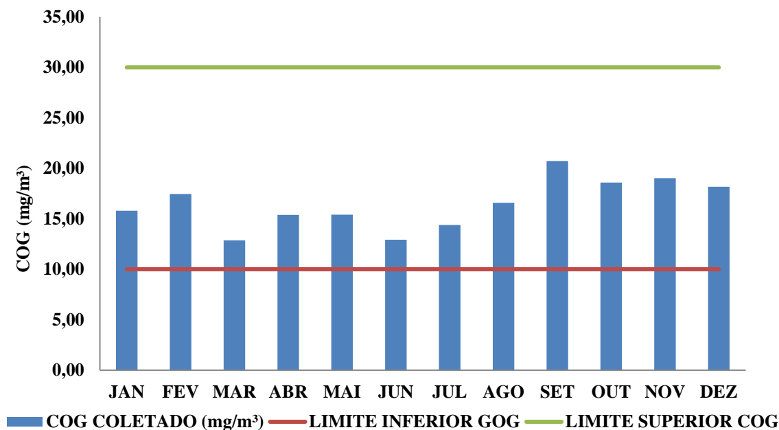
Gráfico 10 - Análise do COG por cromatografia
