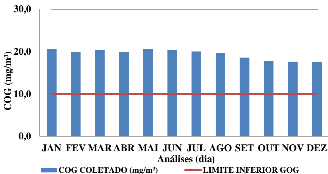
Gráfico 9 - Análise do COG por odorímetro
