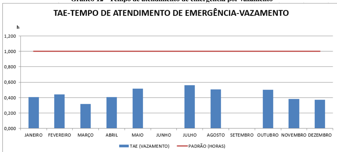
Gráfico 12 - Tempo de atendimento de emergência por vazamento
