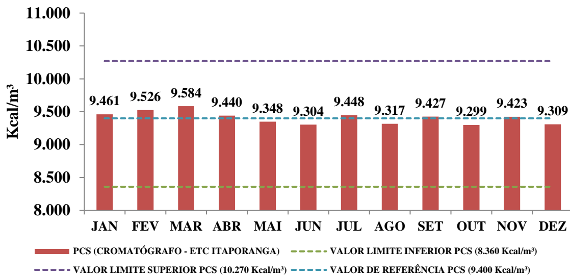
Gráfico 17 - PCS (ETC Itaporanga)
