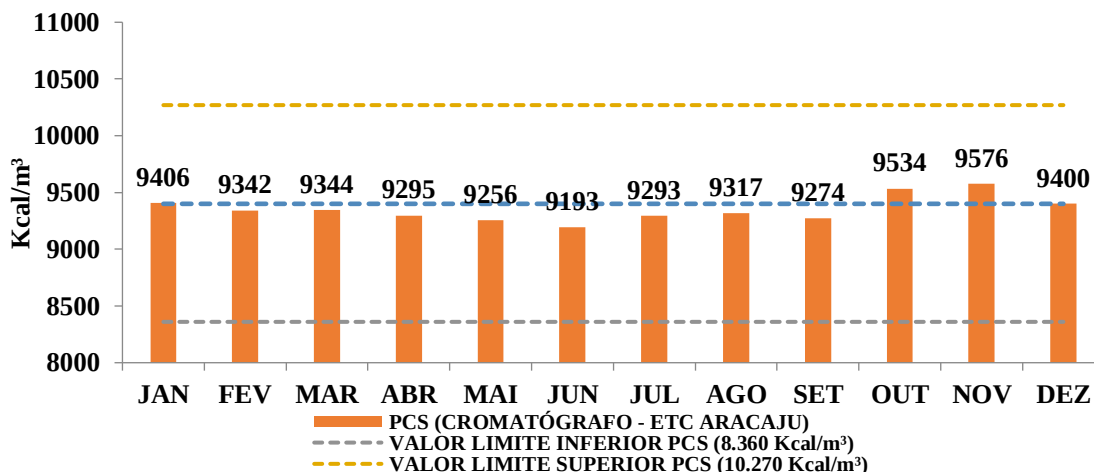
Gráfico 15 - PCS (ETC Aracaju)
