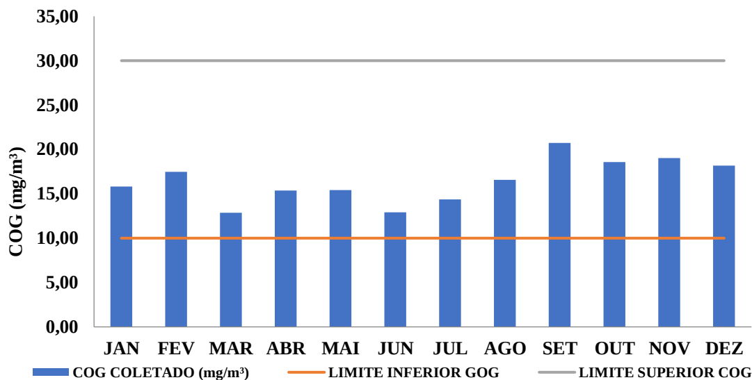
Gráfico 10 - Análise do COG por cromatografia
