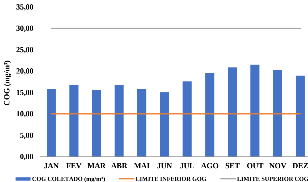
Gráfico 9 - Análise do COG por odorímetro
