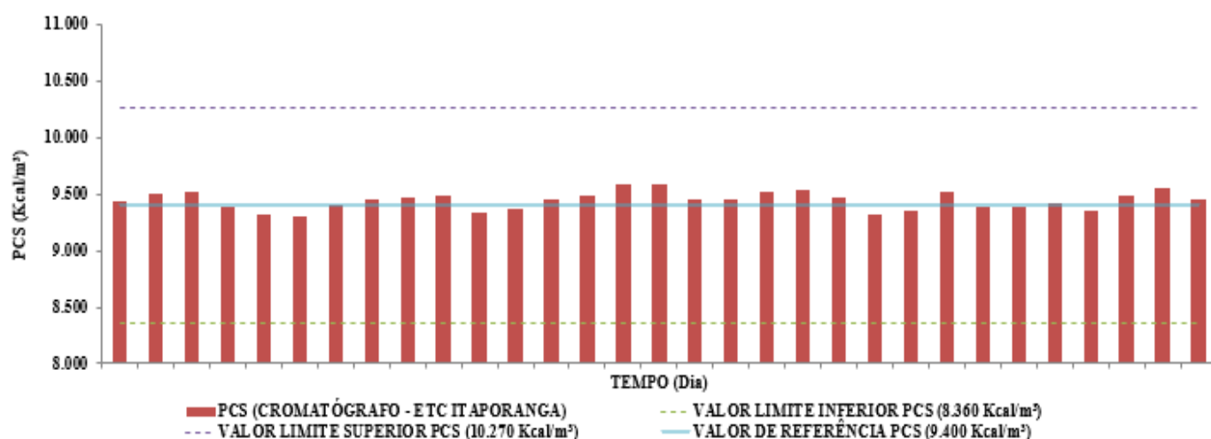
Gráfico 7: PCS ETC Itaporanga
