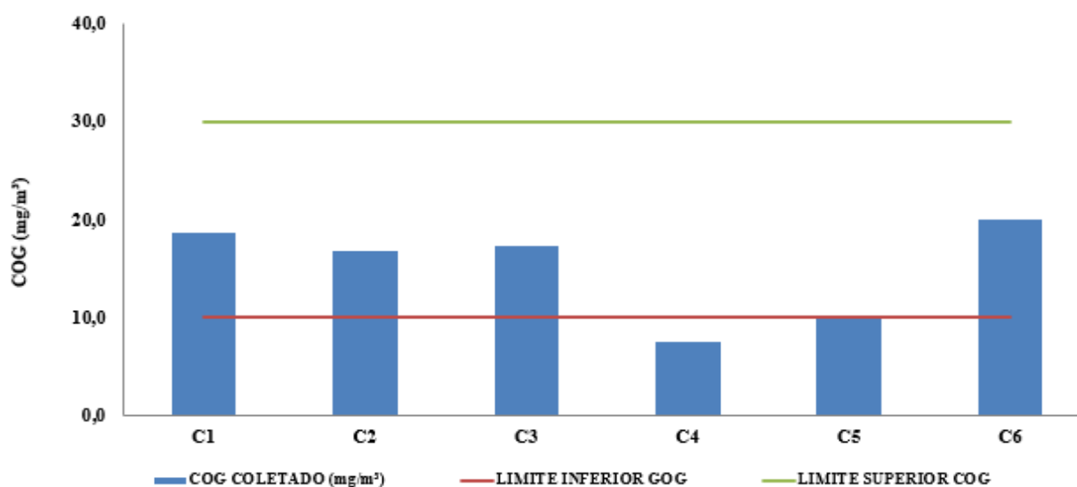
Gráfico 2: Análise Cromatográfica (COG)
