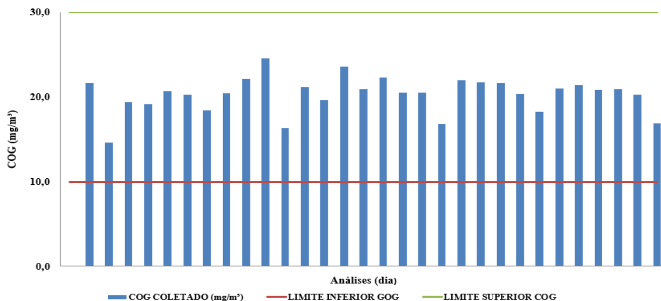
Gráfico 1: Análise por Odorímetro (COG)
