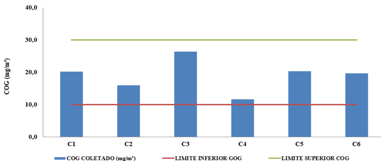
Gráfico 2: Análise Cromatográfica (COG)
