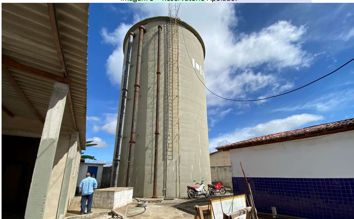
Imagem 3 – Reservatório Apoiado.
