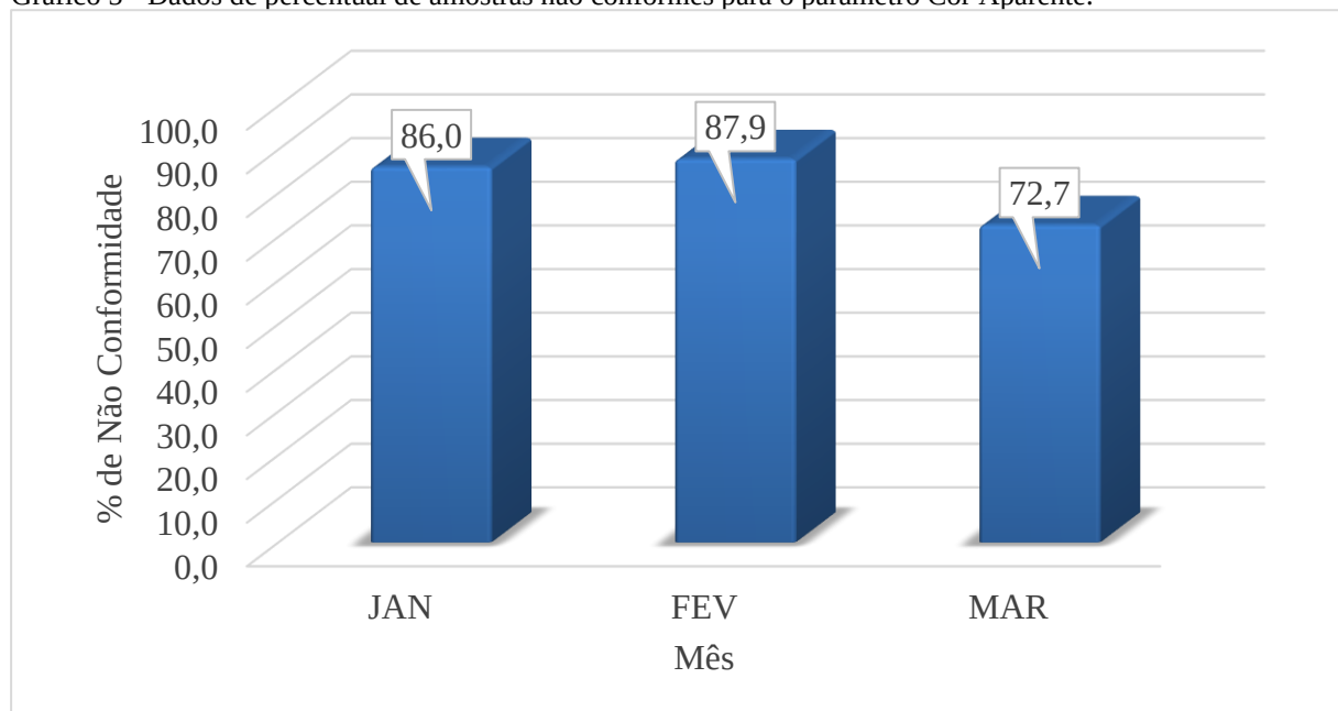
Gráfico 5 - Dados de percentual de amostras não conformes para o parâmetro Cor Aparente.
