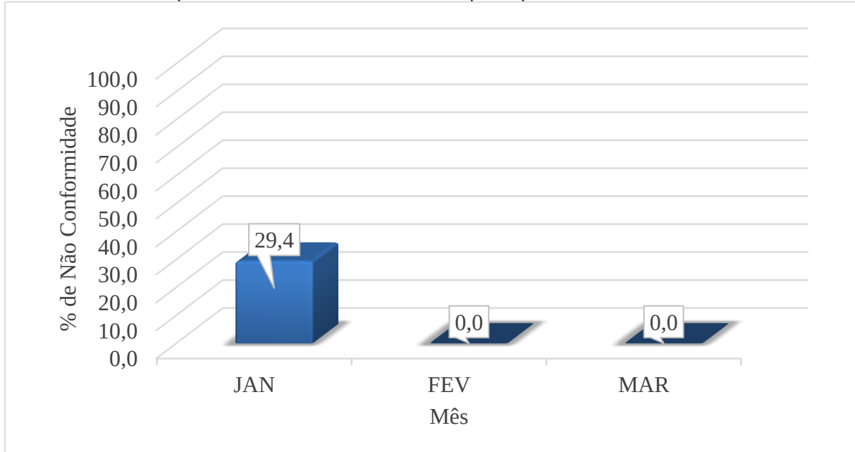
Gráfico 10 - Dados de percentual de amostras não conformes para o parâmetro de Cloro Residual Livre.
