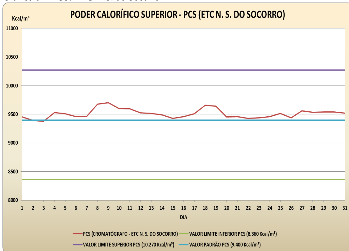
Gráfico 07- PCS: ETC N.S. do Socorro
