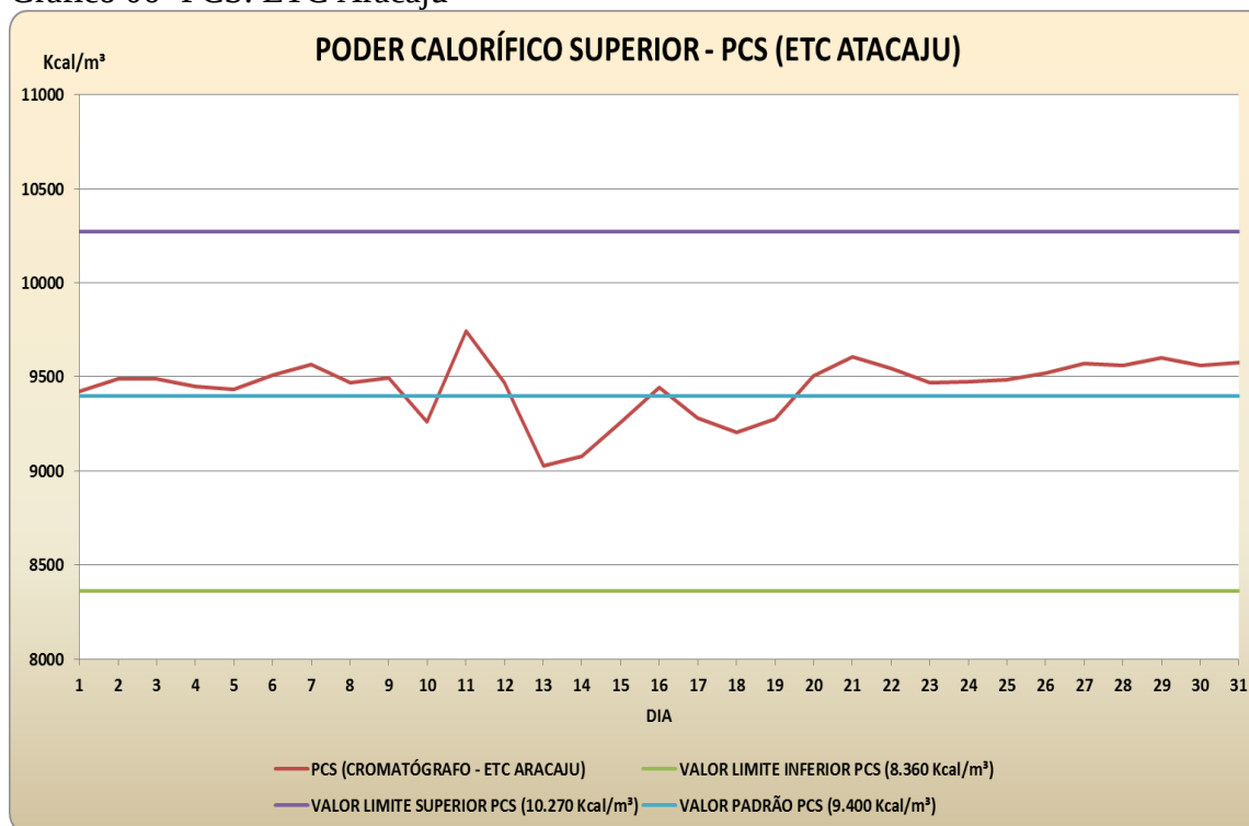
Gráfico 06- PCS: ETC Aracaju
