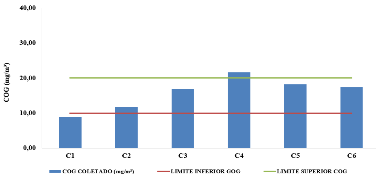
Gráfico 2: Análise Cromatográfica (COG)
