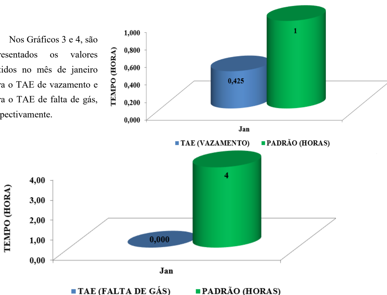
Gráfico 4: TAE Falta de Gás Registrado x TAE Padrão
