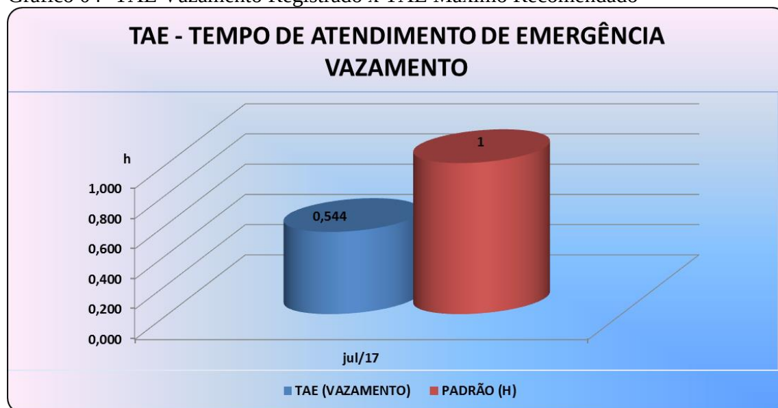
Gráfico 04- TAE Vazamento Registrado x TAE Máximo Recomendado
