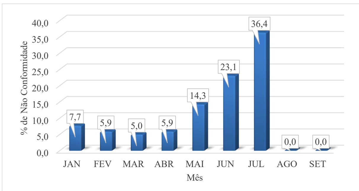
Gráfico 21 - Dados de percentual de amostras não conformes para o parâmetro de Turbidez.
