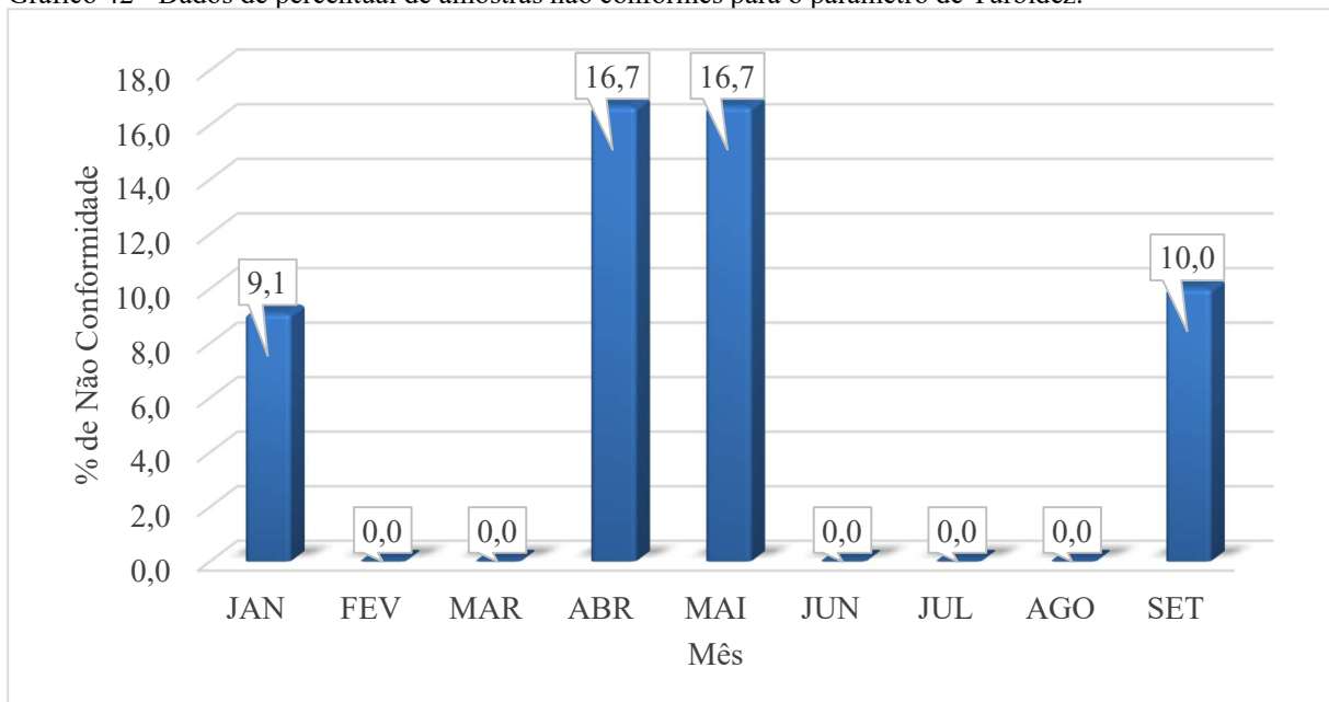
Gráfico 42 - Dados de percentual de amostras não conformes para o parâmetro de Turbidez.
