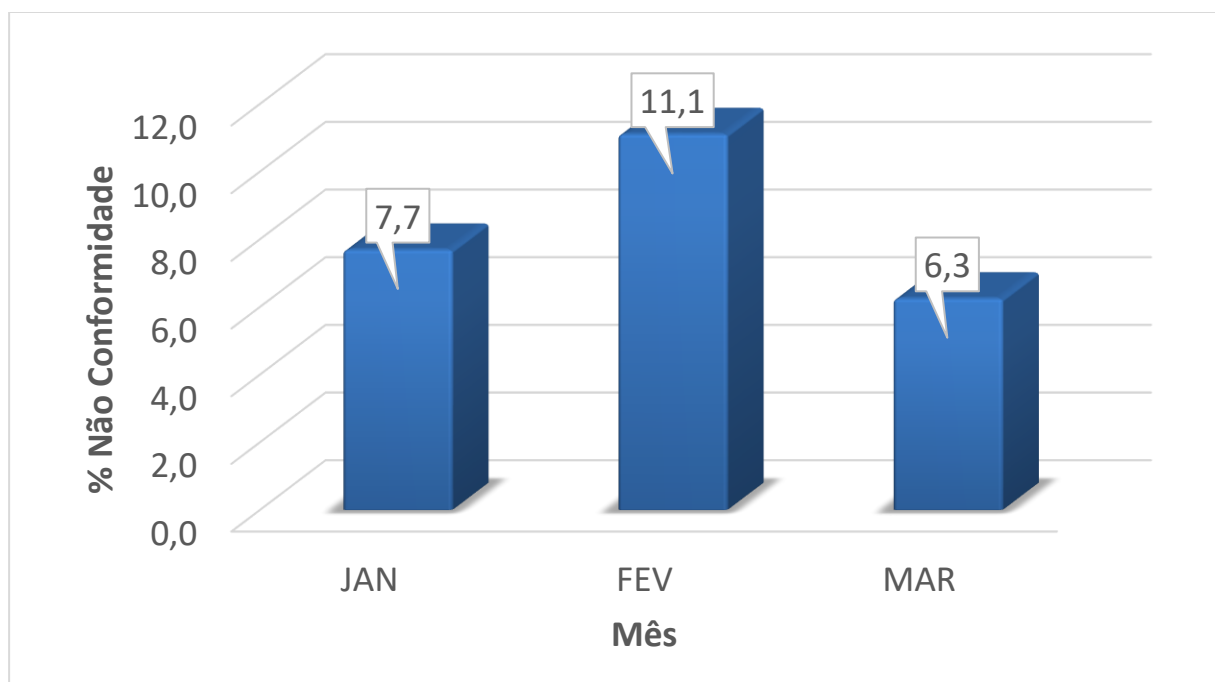
Gráfico 45 - Dados de percentual de amostras não conformes para o parâmetro de Turbidez. FONTE: Adaptado da DESO, 2021.
