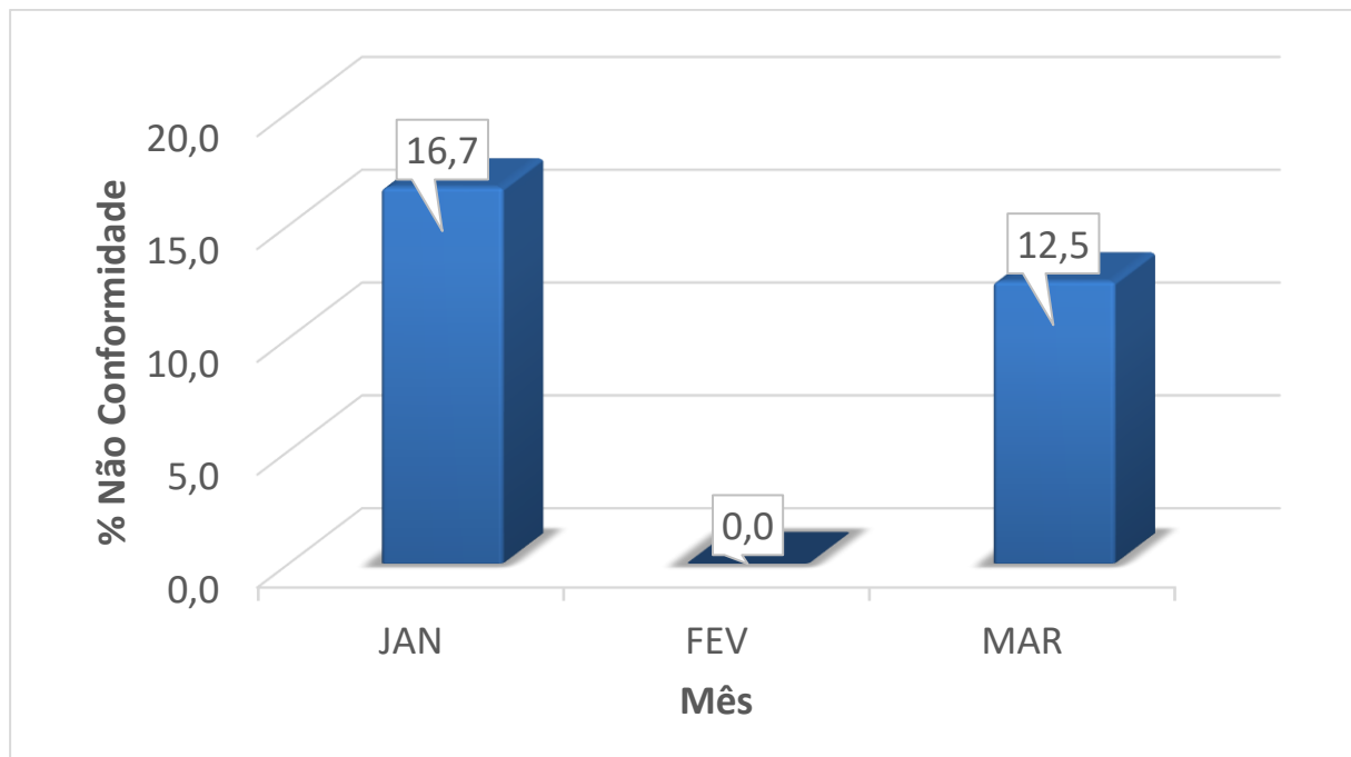
Gráfico 16 - Dados de percentual de amostras não conformes para o parâmetro de Cloro Residual Livre. FONTE: Adaptado da DESO, 2021.
