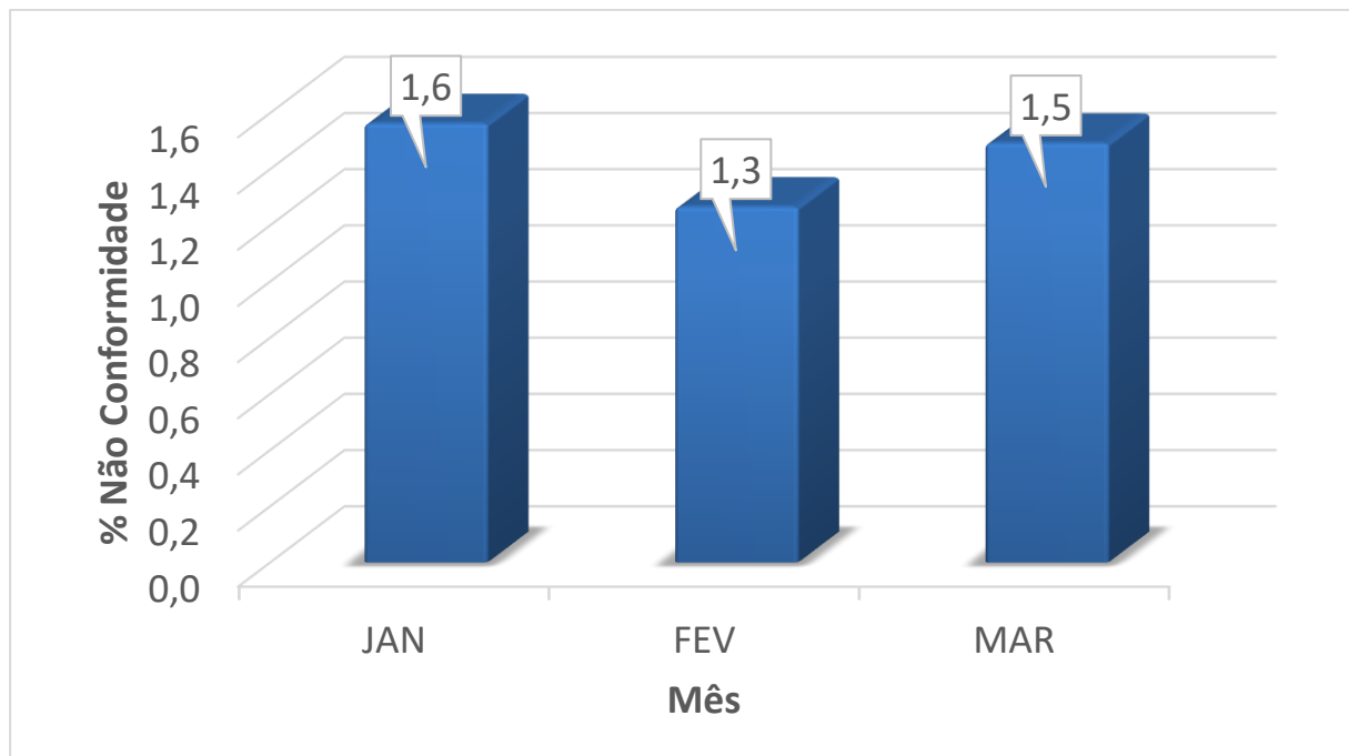
Gráfico 10 - Dados de percentual de amostras não conformes para o parâmetro de Cloro Residual Livre. FONTE: Adaptado da DESO, 2021.
