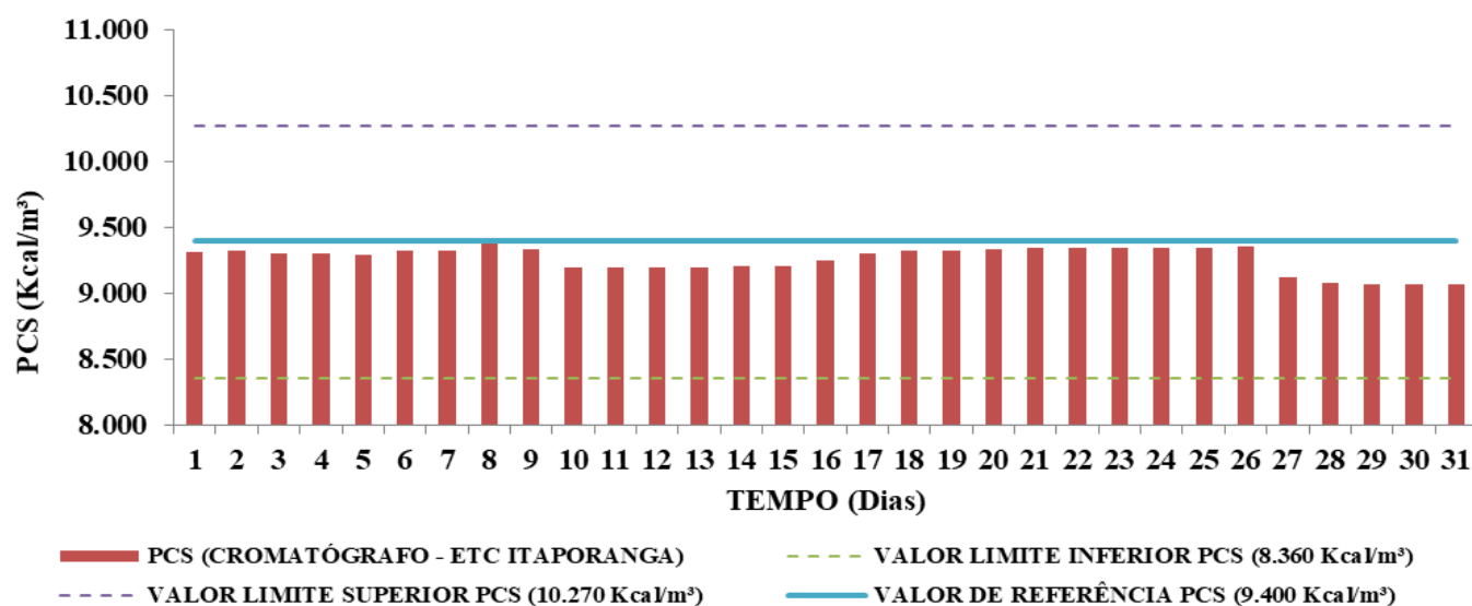
Gráfico 6: PCS ETC Itaporanga
