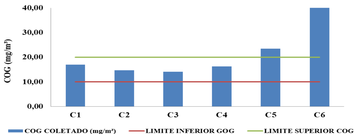
Gráfico 2: Análise Cromatográfica (COG)
