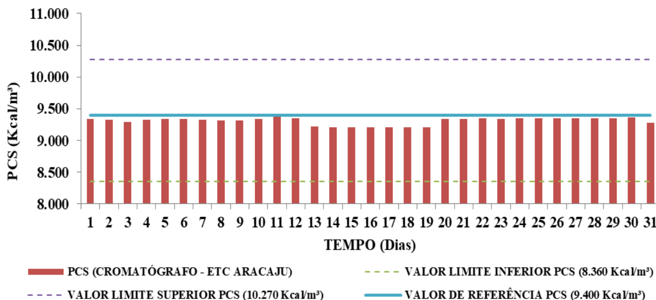
Gráfico 4: PCS ETC Aracaju
