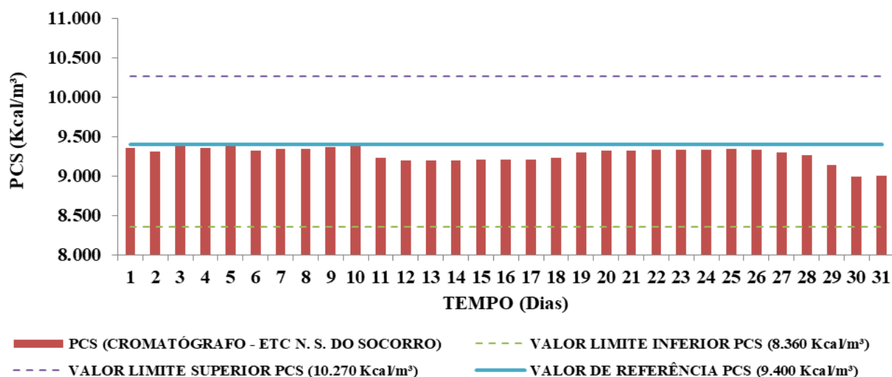
Gráfico 5: PCS ETC Nossa Senhora do Socorro
