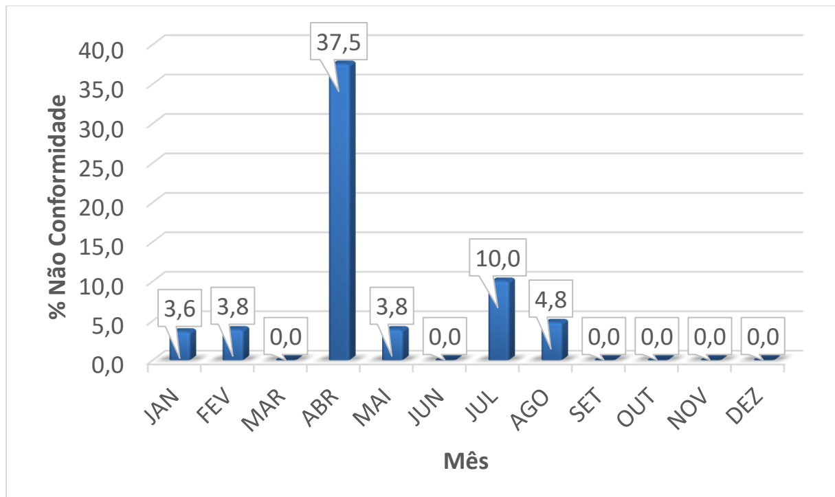
Gráfico 34 - Dados de percentual de amostras não conformes para o parâmetro de Cloro Residual Livre. FONTE: Adaptado da DESO, 2020.
