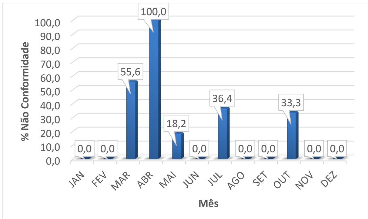
Gráfico 58 - Dados de percentual de amostras não conformes para o parâmetro de Cloro Residual Livre. FONTE: Adaptado da DESO, 2020.
