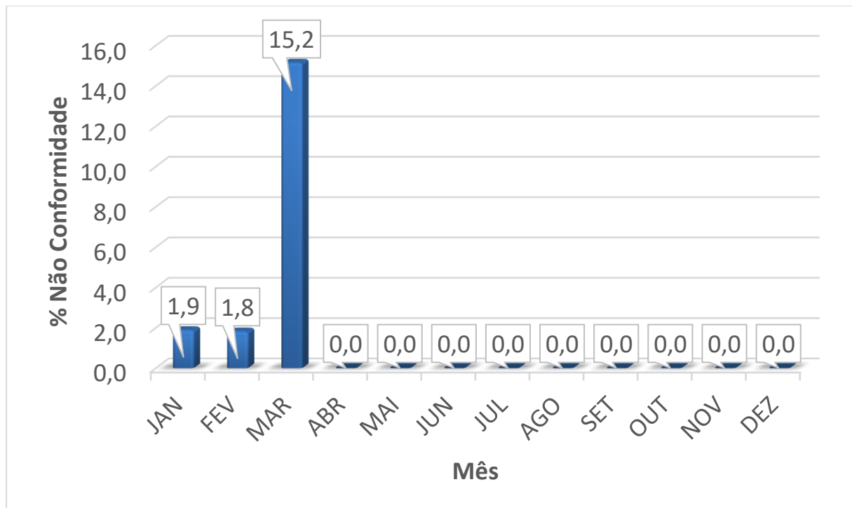
Gráfico 55 - Dados de percentual de amostras não conformes para o parâmetro de Cloro Residual Livre. FONTE: Adaptado da DESO, 2020.
