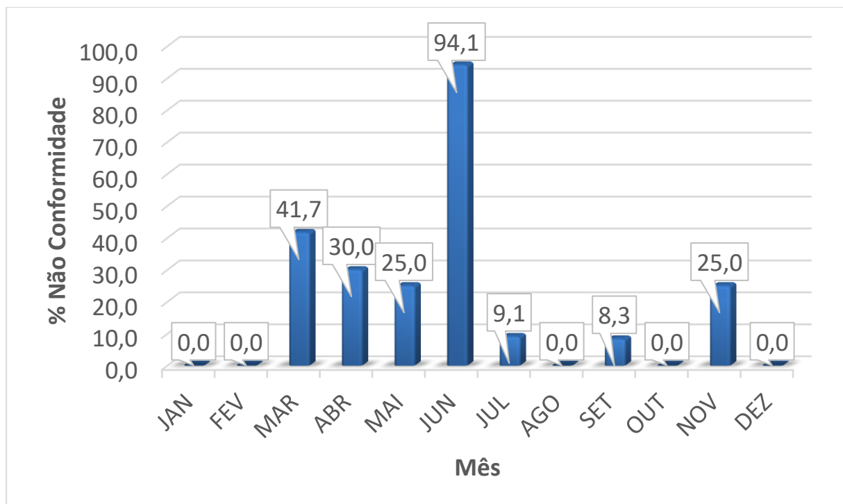
Gráfico 19 - Dados de percentual de amostras não conformes para o parâmetro de Cloro Residual Livre. FONTE: Adaptado da DESO, 2020.
