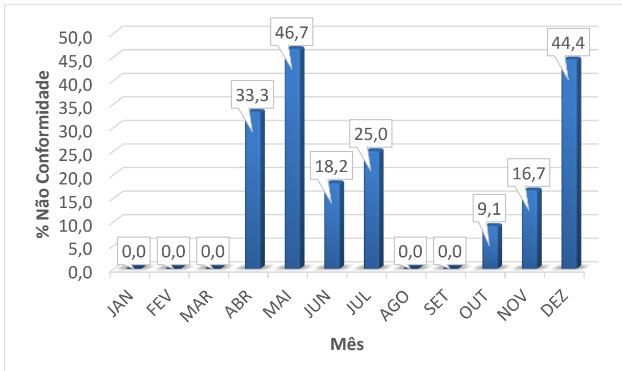
Gráfico 49 - Dados de percentual de amostras não conformes para o parâmetro de Cloro Residual Livre. FONTE: Adaptado da DESO, 2020.
