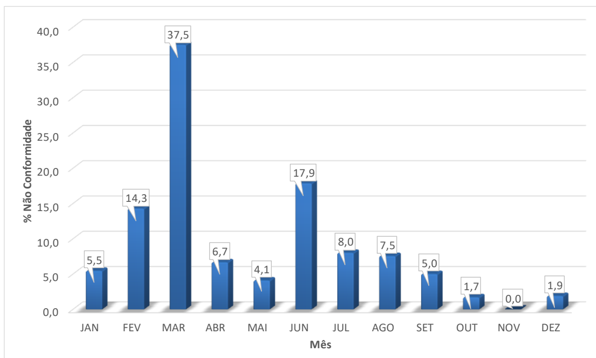
Gráfico 42 - Dados de percentual de amostras não conformes para o parâmetro de Turbidez. FONTE: Adaptado da DESO, 2020.
