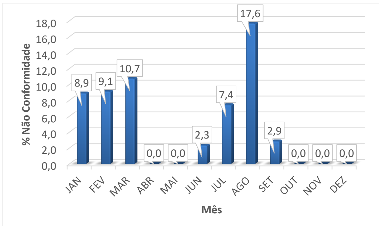
Gráfico 10 - Dados de percentual de amostras não conformes para o parâmetro de Cloro Residual Livre. FONTE: Adaptado da DESO, 2020.
