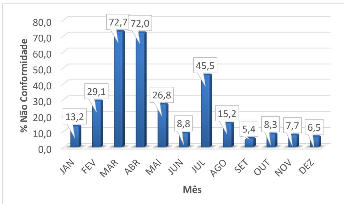
Gráfico 57 - Dados de percentual de amostras não conformes para o parâmetro de Turbidez. FONTE: Adaptado da DESO, 2020.
