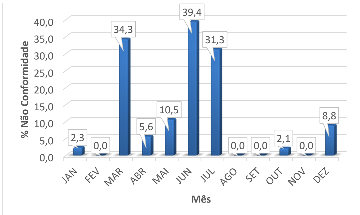
Gráfico 4 - Dados de percentual de amostras não conformes para o parâmetro de Cloro Residual Livre. FONTE: Adaptado da DESO, 2020.
