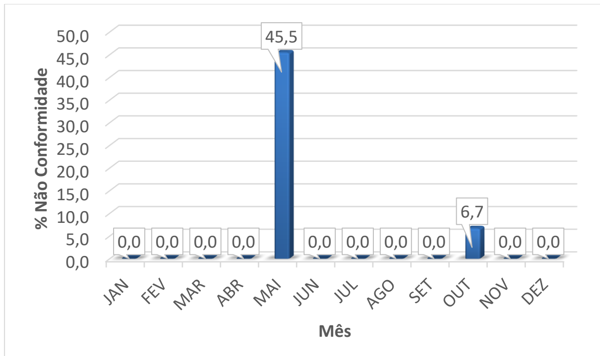
Gráfico 7 - Dados de percentual de amostras não conformes para o parâmetro de Cloro Residual Livre. FONTE: Adaptado da DESO, 2020.
