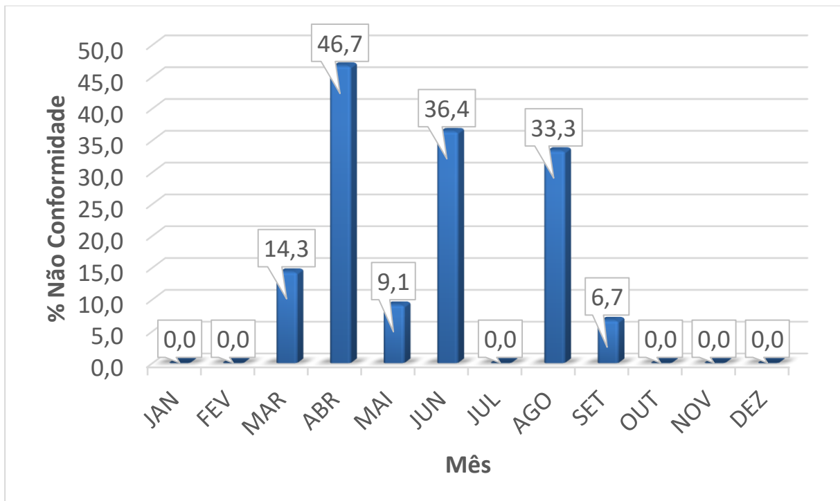
Gráfico 46 - Dados de percentual de amostras não conformes para o parâmetro de Cloro Residual Livre. FONTE: Adaptado da DESO, 2020.
