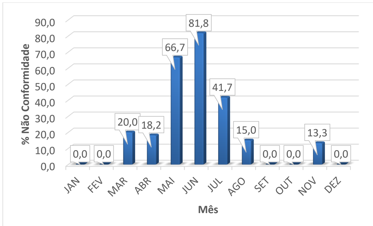
Gráfico 16 - Dados de percentual de amostras não conformes para o parâmetro de Cloro Residual Livre. FONTE: Adaptado da DESO, 2020.
