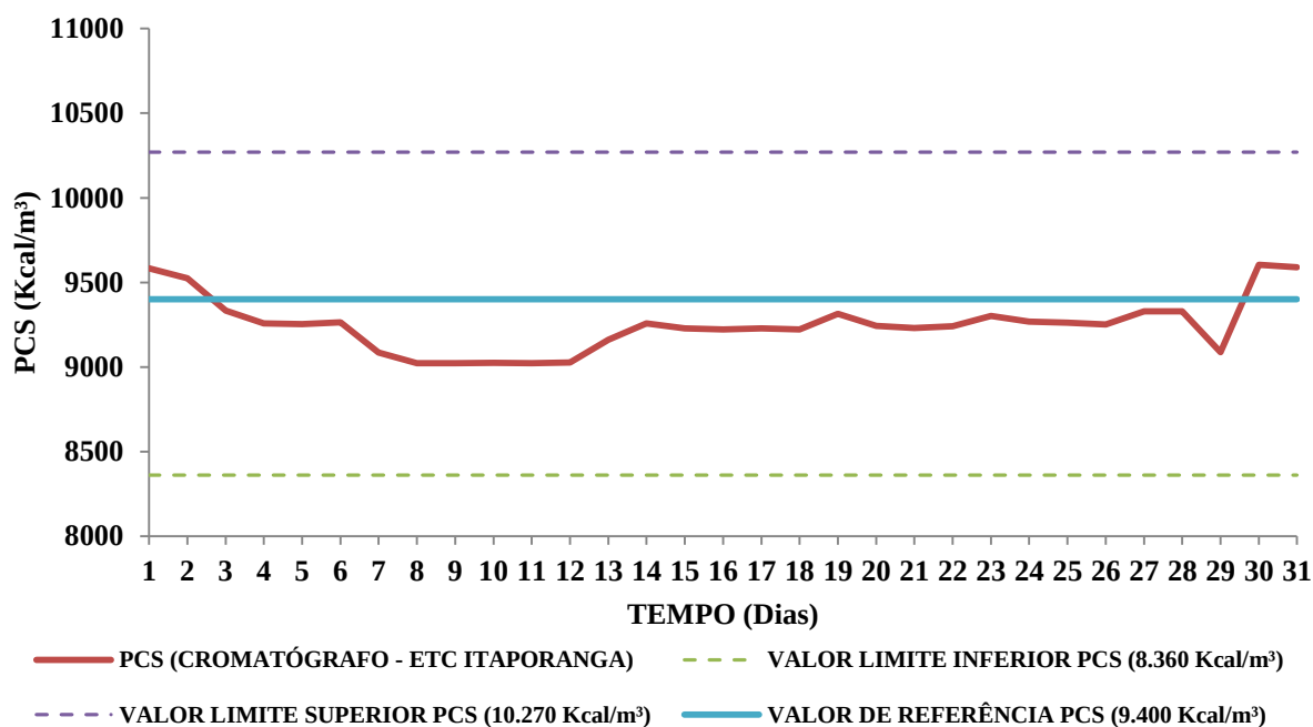
Gráfico 8: PCS ETC Itaporanga
