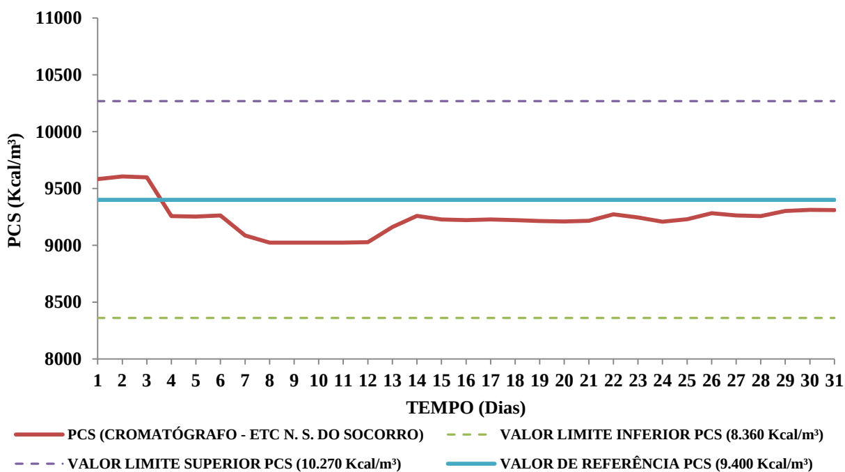
Gráfico 7: PCS ETC Nossa Senhora do Socorro
