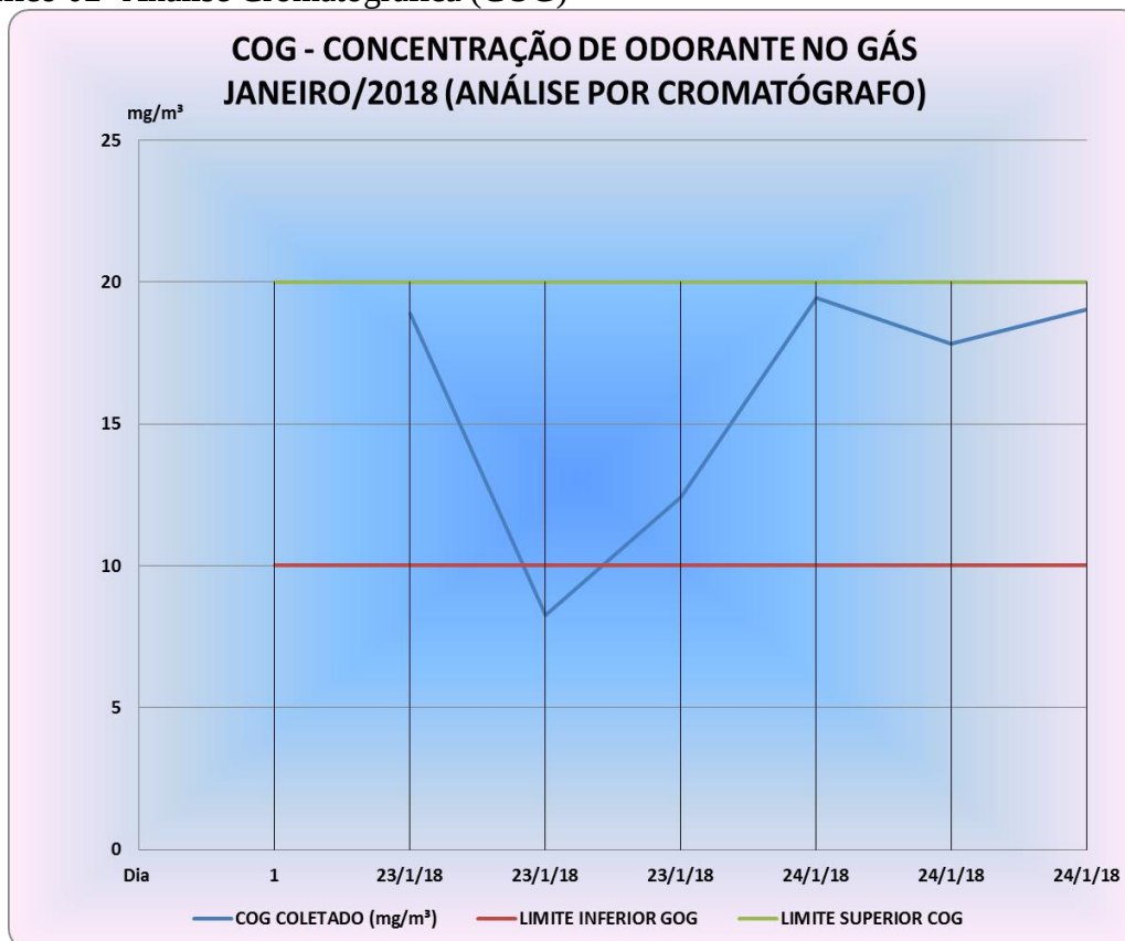
Gráfico 02- Análise Cromatográfica (COG)
