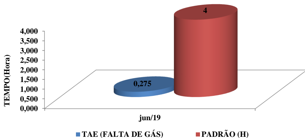
Gráfico 05: TAE Falta de Gás Registrado x TAE Máximo Recomendado
